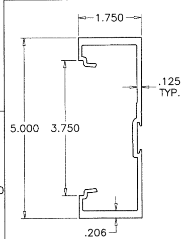
E07 DOOR MULLION
