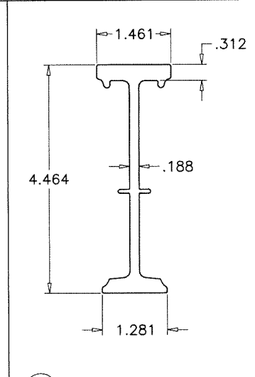
E06 STIFFENER
